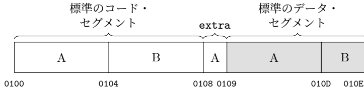
図 24.1: tanren a b のメモリ。それぞれの箱が、セグメントの中の 1 つのモジュールの部分です。網掛けの箱はデータです。
