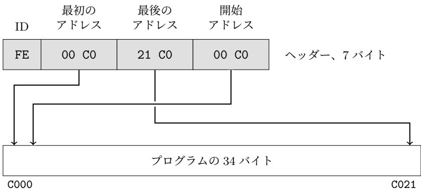
図 26.1: HELLOB.BIN の BLOAD ヘッダーと、そこに入っている 3 つのアドレス。
