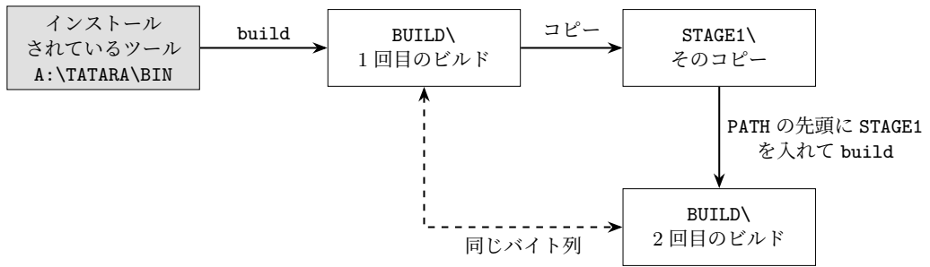
図 35.3: ツールを 2 回ビルドする。2 回目は、1 回目のビルドで作ったツールを使う。
