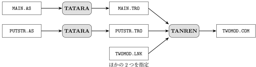
図 28.1: BUILD.BAT が TWOMOD.COM を作る流れ。
