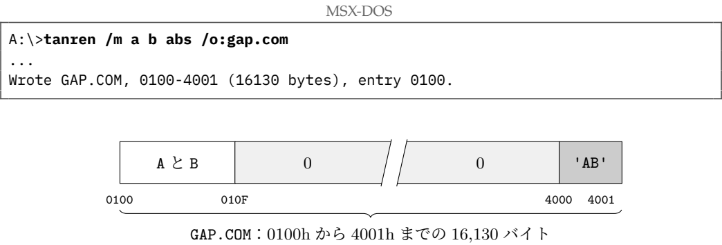
図 24.3: コードよりずっと上にあるアブソリュート・セグメント。間の部分も 0 としてファイルに入ります。
