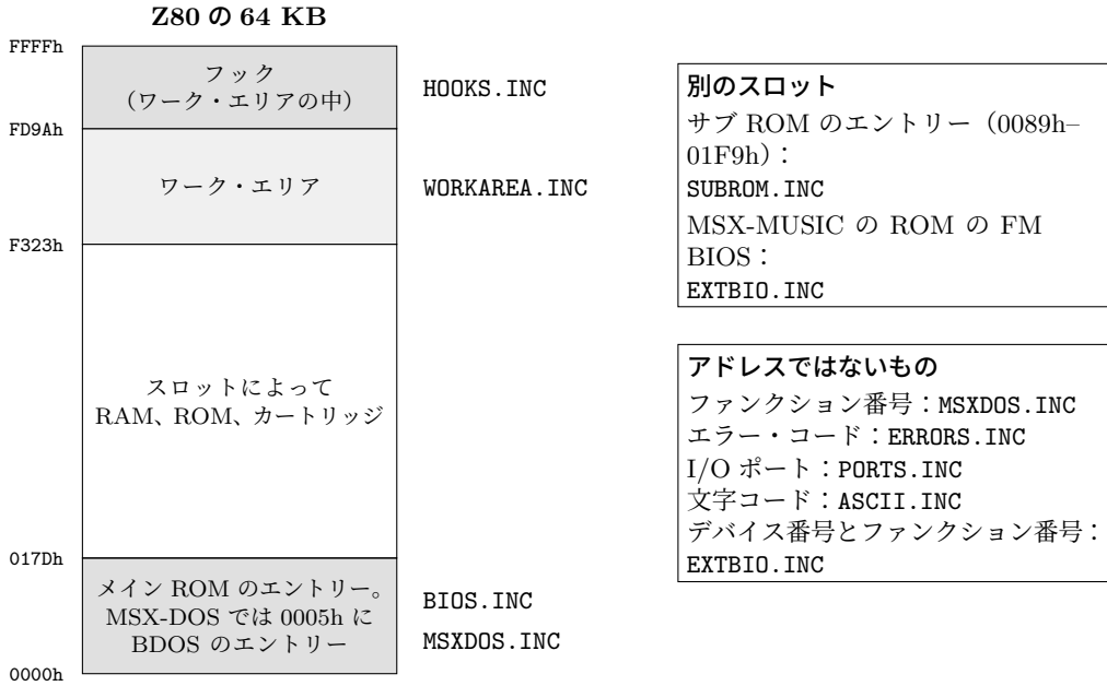
図 K.1: インクルード・ファイルが名前を付けているアドレスの位置
