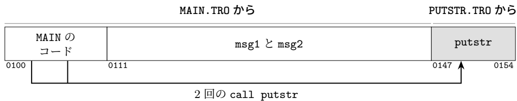
図 28.2: メモリの中の TWOMOD.COM。MAIN の 2 つの呼び出しは、どちらも 0147h の putstr に行きます。
