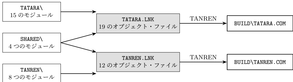
27のソース、27のオブジェクト・ファイル
