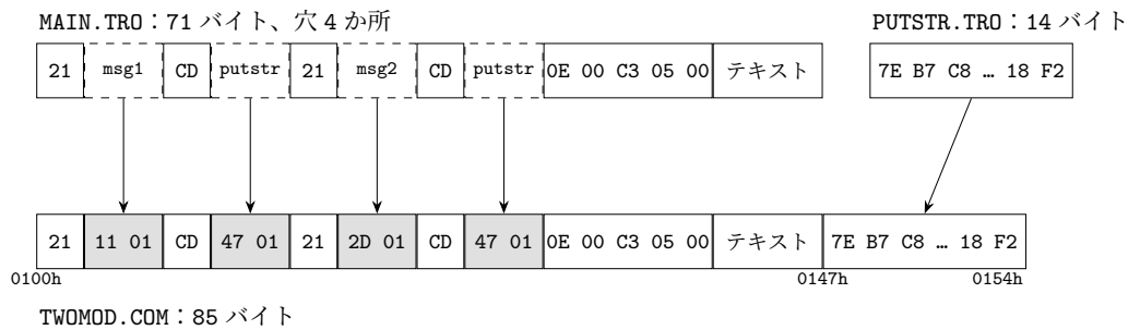
図 2.2: MAIN.TRO と PUTSTR.TRO をリンクして TWOMOD.COM を作る
