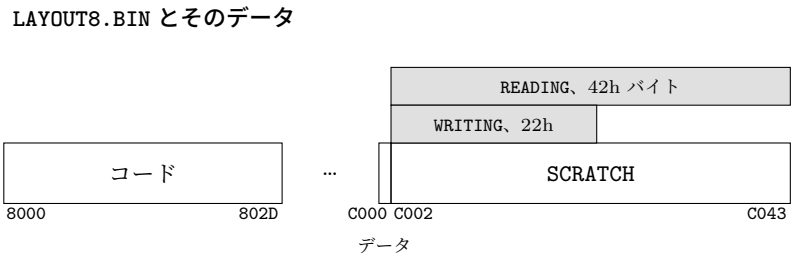
図 29.1: 0100h でリンクした LAYOUT と、コードを 8000h、データを C000h にしてリンクした LAYOUT。どちらも、SCRATCH の 2 つのグループは同じアドレスから始まります。
