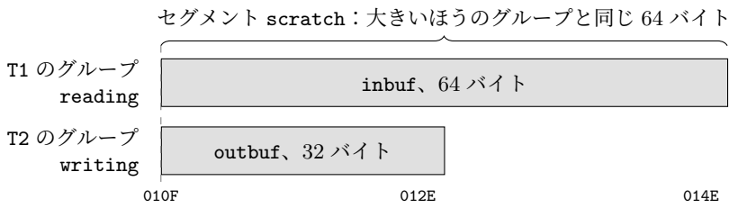
図 24.2: 2つのモジュールから加えたトランジェント・セグメント scratch の2つのグループが、同じアドレスにある様子
