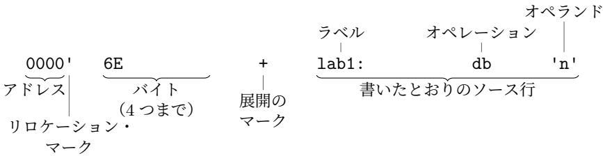
図 18.1: リスティングの1行の欄
