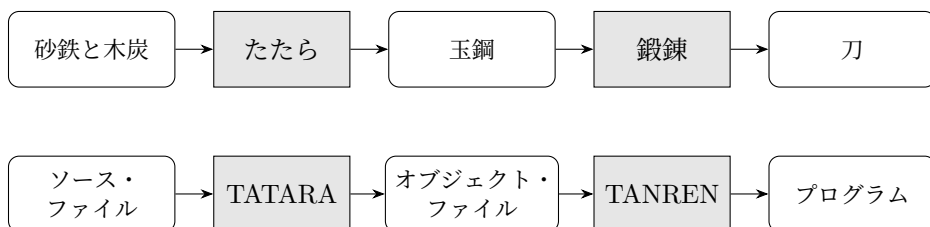
図 1.1: 原料から完成した刀へ、ソース・ファイルから完成したプログラムへ
