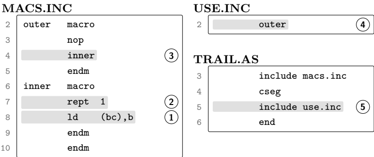
図 20.1: メッセージと経路の各行と、それが示すソースの行
