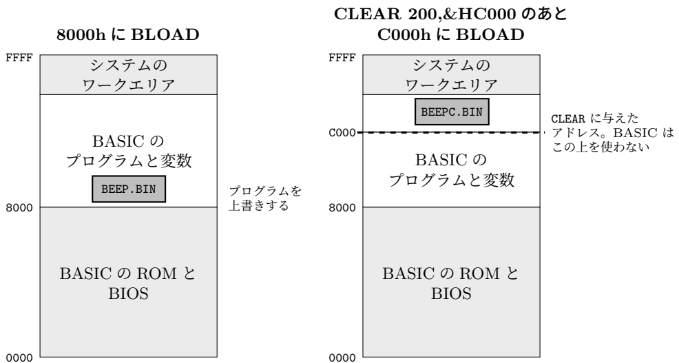
図 32.1: MSX-BASIC のメモリ。ファイルを 8000h に置いた場合と、C000h に置いた場合。
