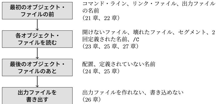
図 27.1: リンクの段階と、それぞれの段階で TANREN が見つける誤り。
