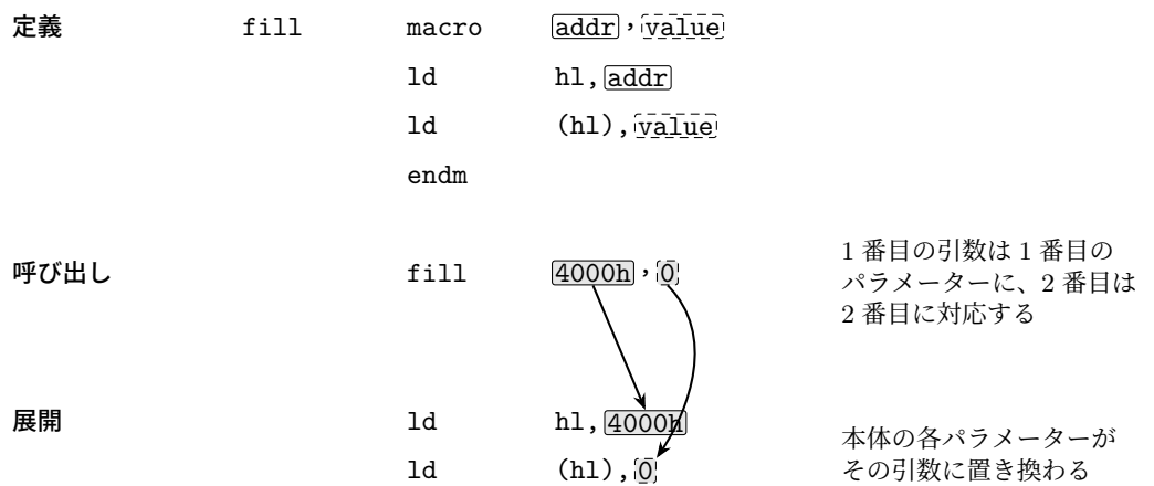
図 16.1: マクロの定義、その使用、そして展開
