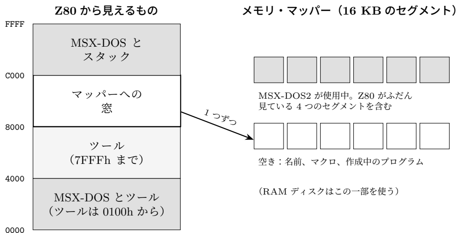
図 G.1: TATARA や TANREN が動いている間の Z80 の 64 KB と、窓の後ろにあるマップパーのセグメント
