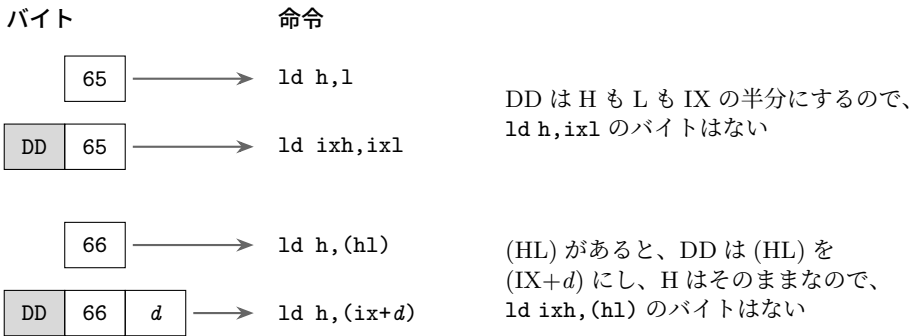
図 9.1: プレフィックスは命令全体にかかる。DD が 2 つの命令にどう働くか
