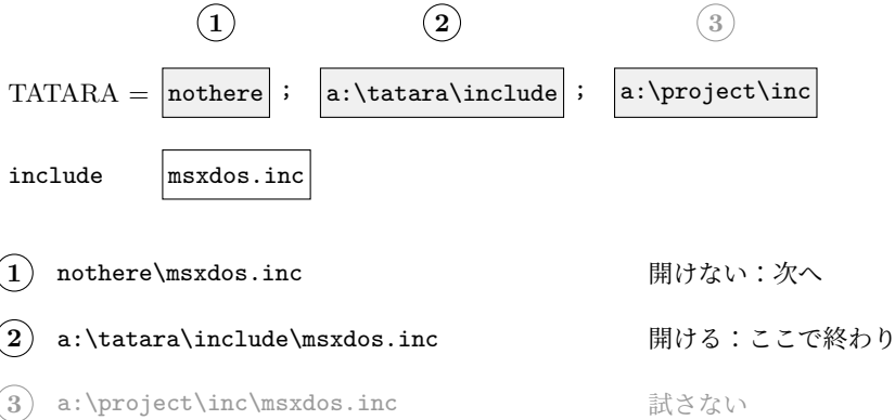
図 I.1: TATARA の値と INCLUDE の行の名前から、試す名前ができる様子（試す順）
