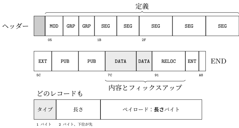
図 F.1: レコードの並びとしての OBJ.TRO と、1 つのレコードの形。箱の幅はバイト数を表す。
